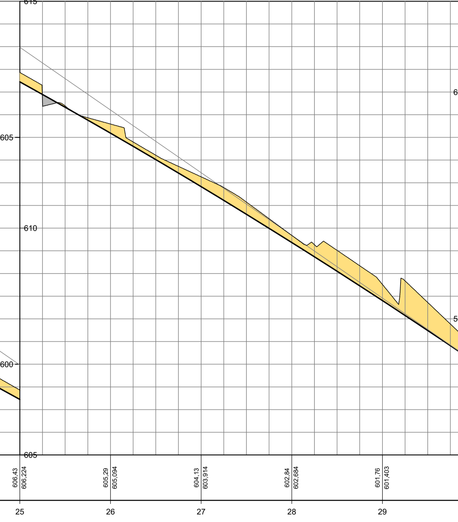
PERFIL ALINHAMENTO - 08
