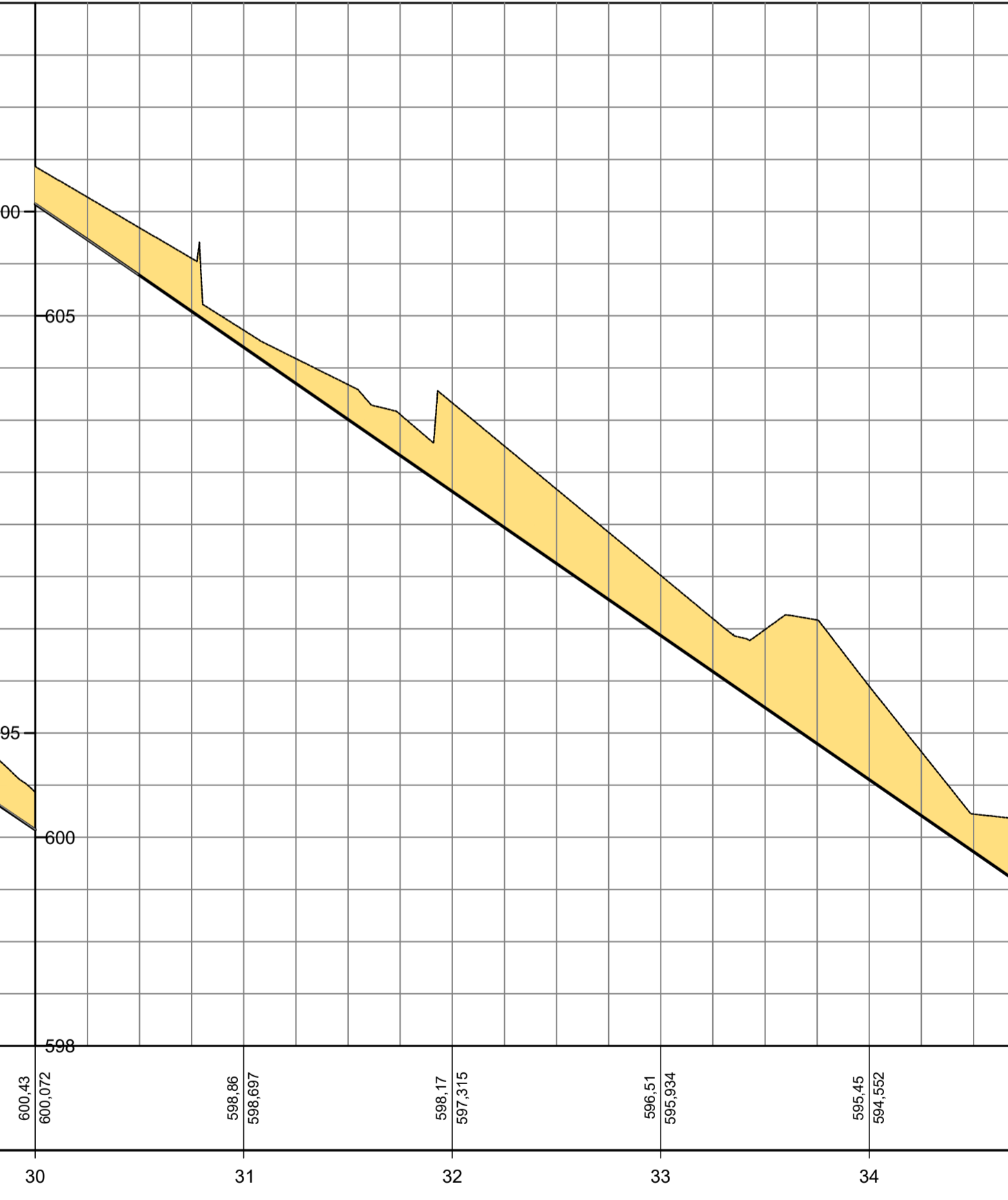
PERFIL ALINHAMENTO - 08
