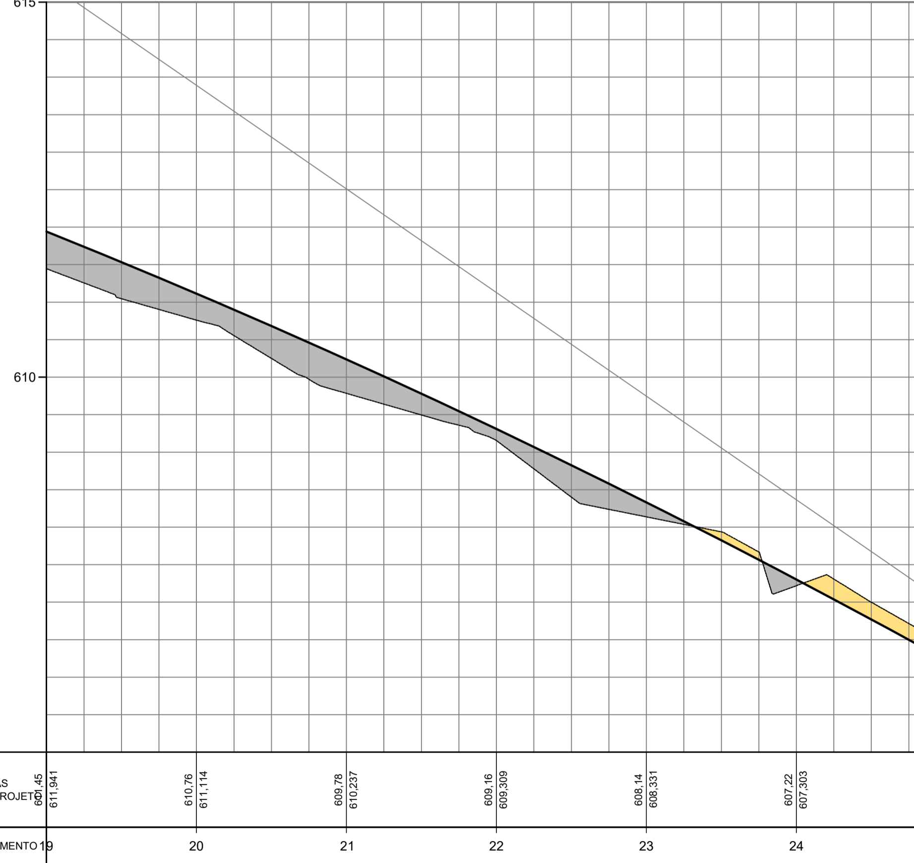
PERFIL ALINHAMENTO - 08
