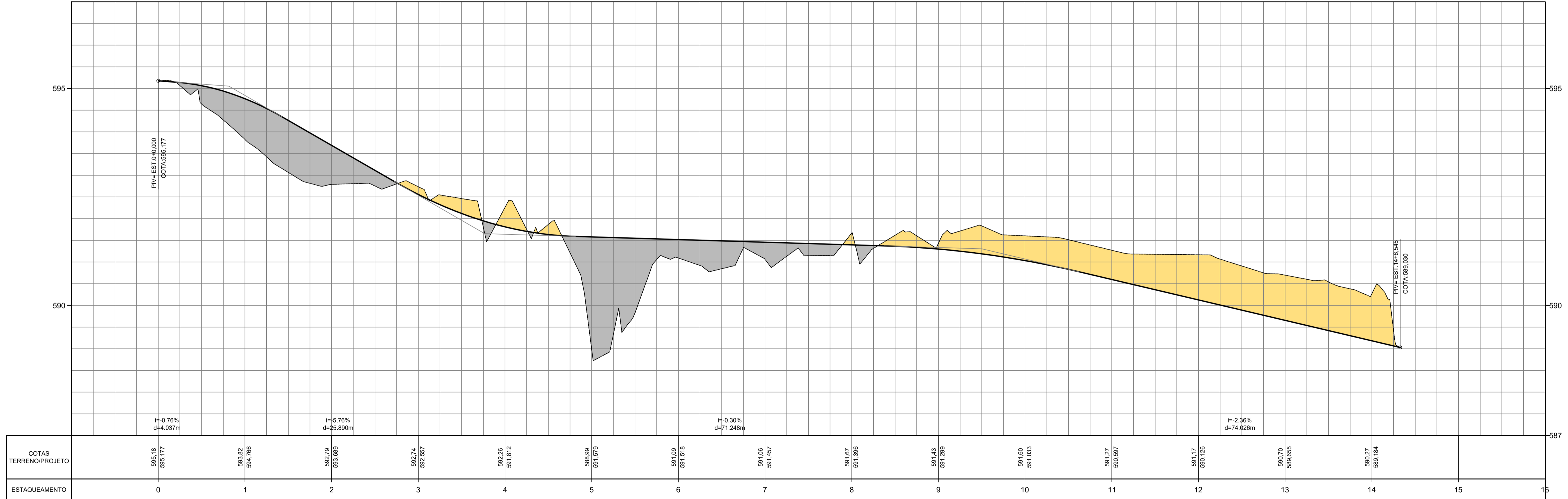
PERFIL ALINHAMENTO - 04
