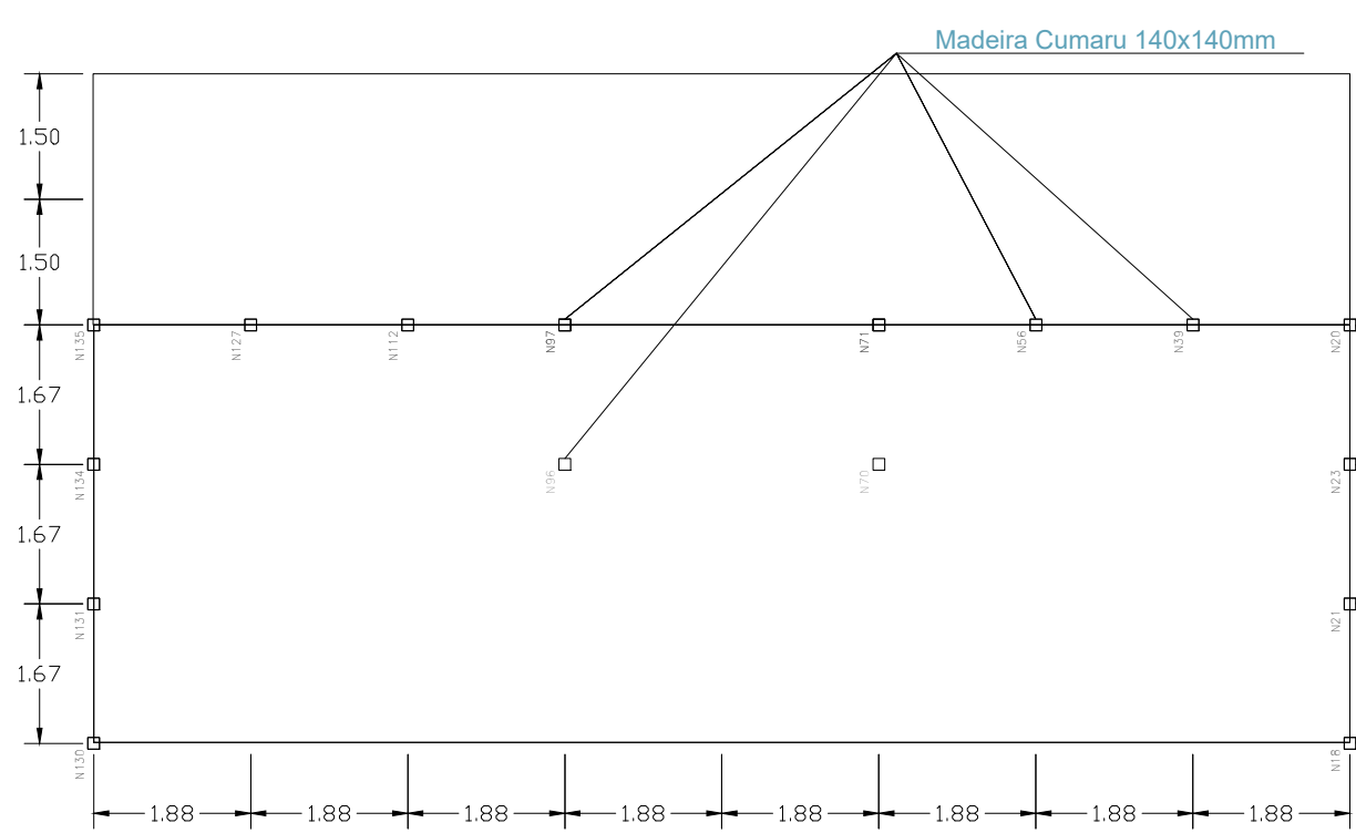
Localização dos Pilares - GUARDA CORPO escala: 1:100
