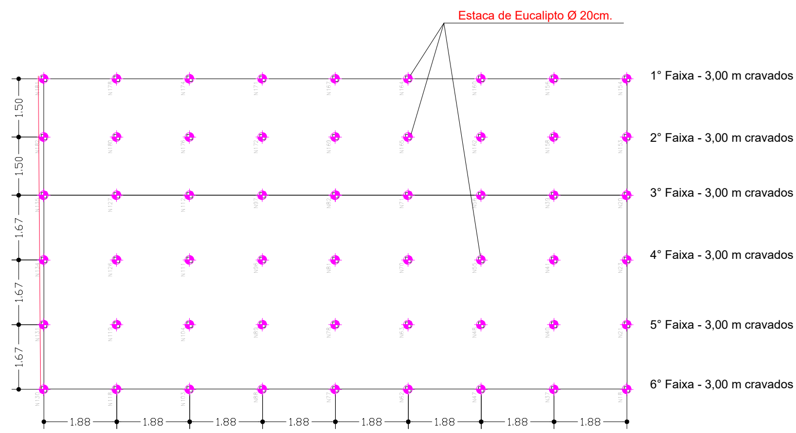
Localização das Estacas de Fundação escala: 1:100
