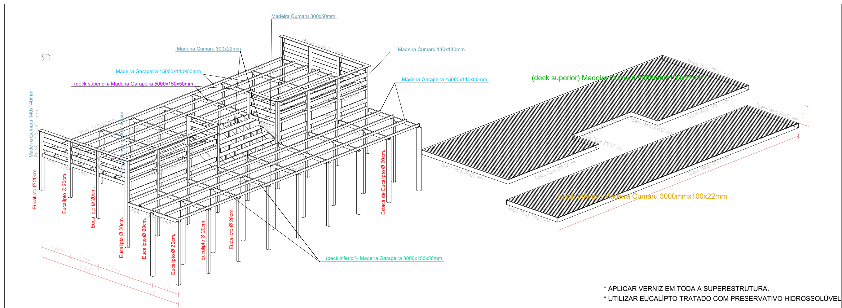
DETALHE 02
