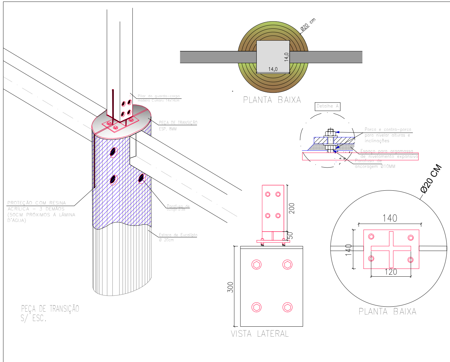
DETALHE 02
