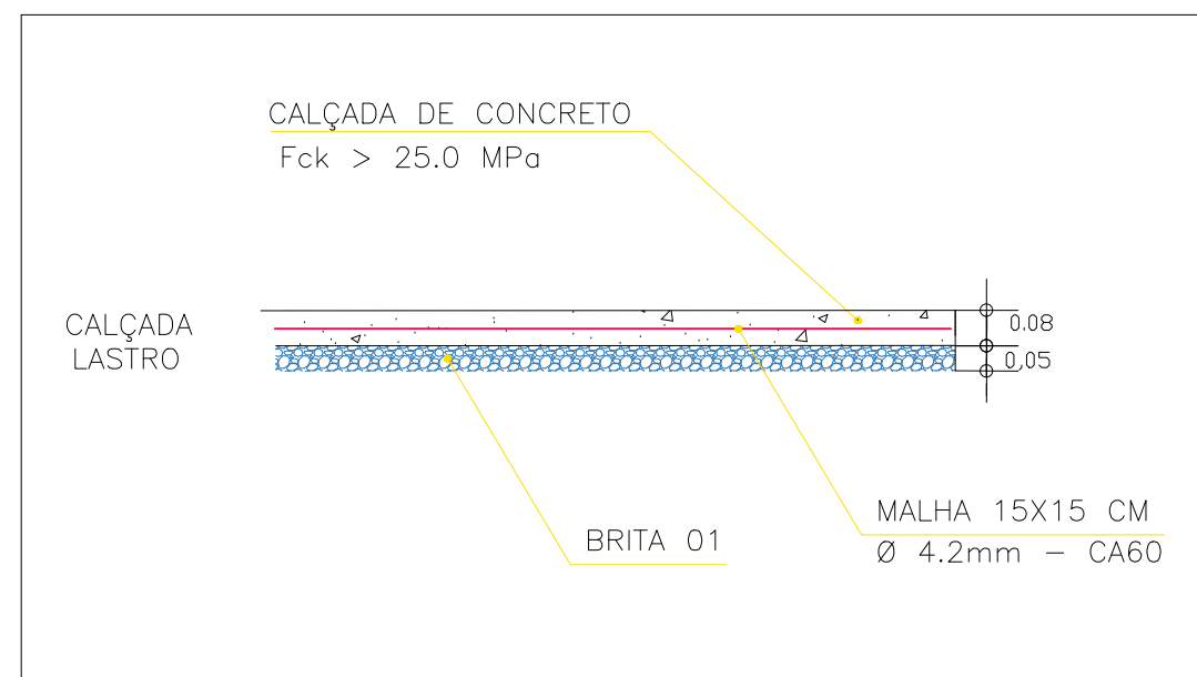
DETALHE 02
